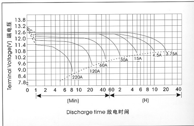
Discharge Curve 77 °F(25 °C)* 放电曲线
